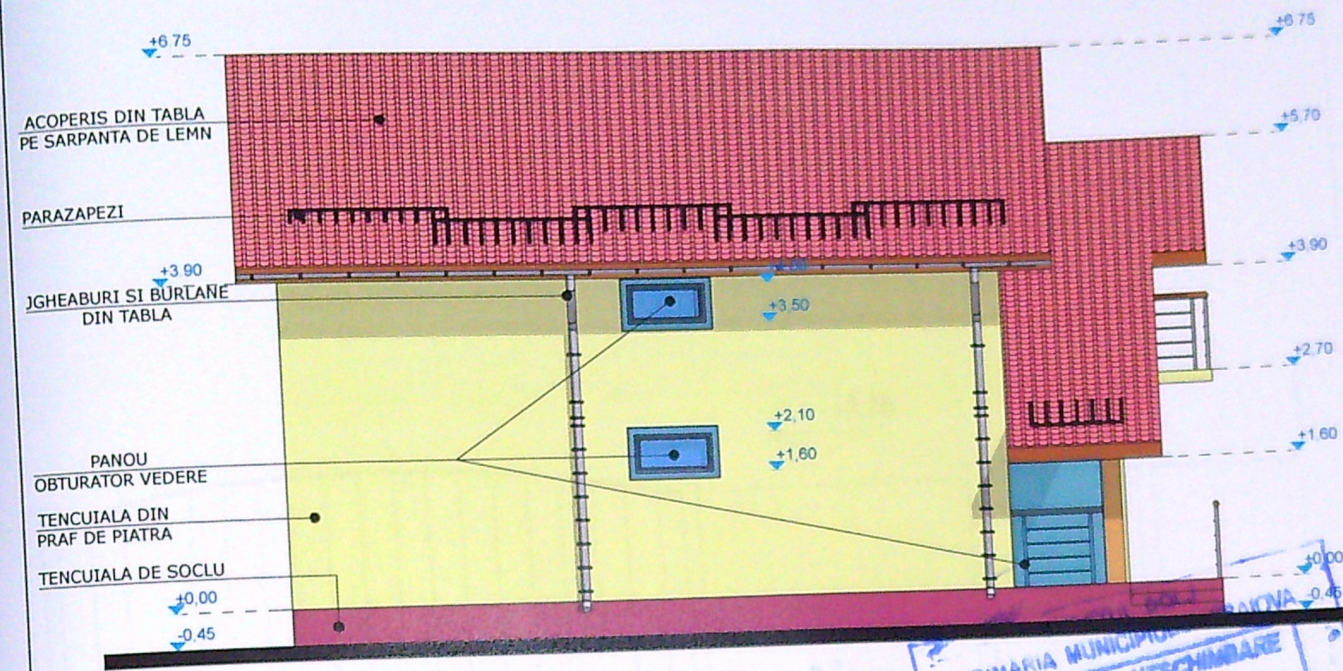
FATADA VEST SCARA 1:100
